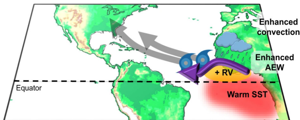
(a) Atlantic Niño
