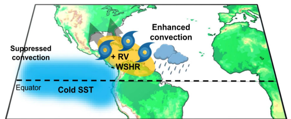
(b) La Niña
