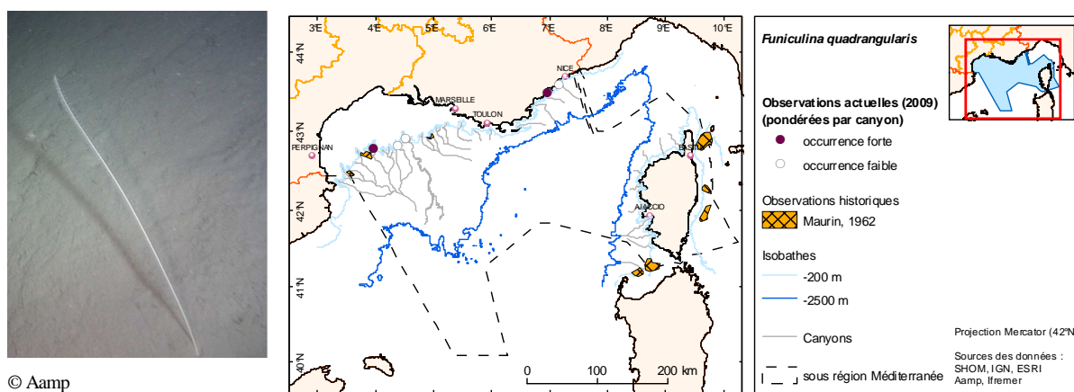
Figure 3 : Carte de localisation des vases molles à Funicula quadrangularis observées pendant la campagne MEDSEACAN 2009 (Aamp/Comex) et dans les données historiques en Méditerranée occidentale. Elles ont probablement été observées pendant la campagne CORSEACAN 2010 (Aamp), mais les vidéos n'ont pas pu être visionnées dans le cadre de l'état initial de la DCSSM.
