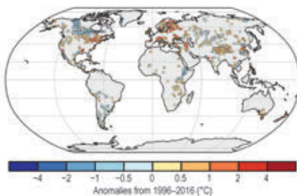
(d) Cool Nights
